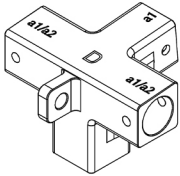
(D) Beveled Right-Angle Cross Connector*2
